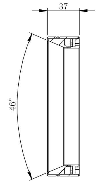
剖面 G-G
