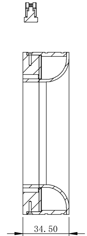
剖面 D-D
