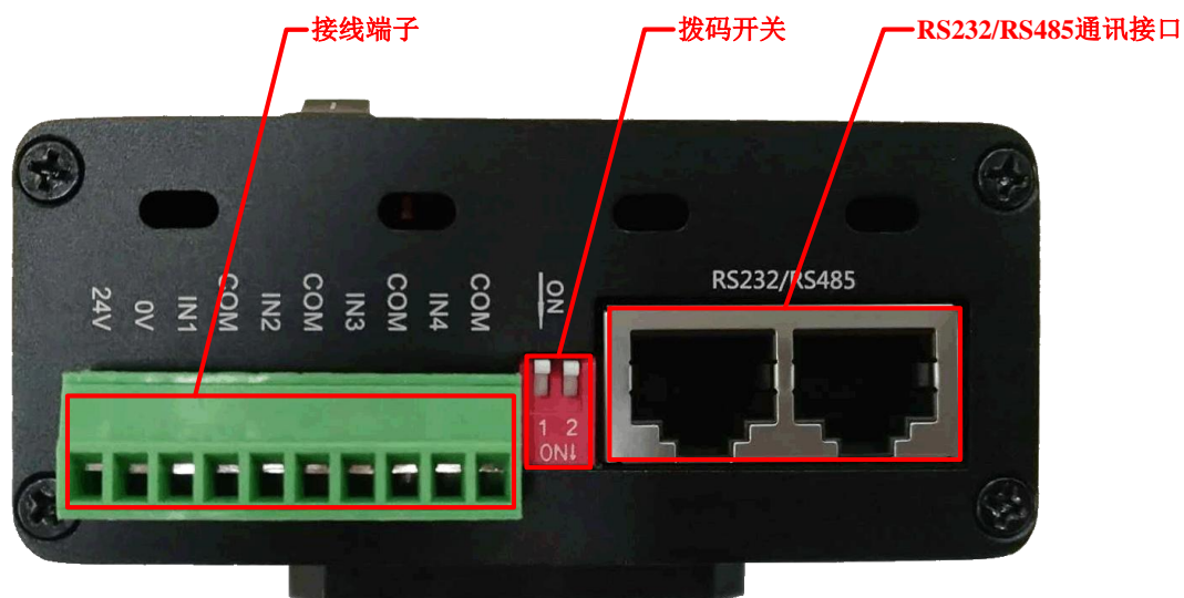
Fig.1 接线端子
