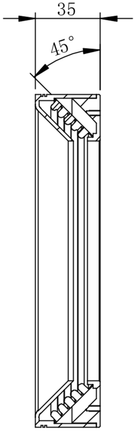
剖面 G-G
