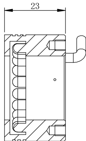
剖面 C-C
