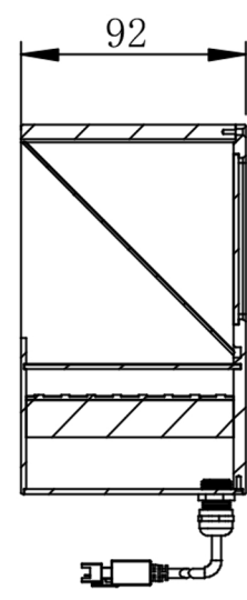
剖面 C-C
