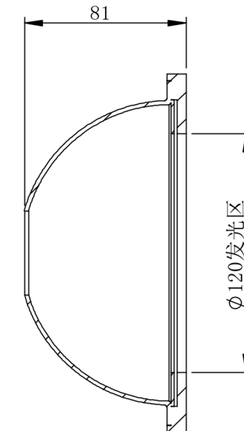
剖面 F-F
