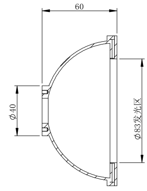
剖面 E-E
